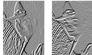
Sx + 128
